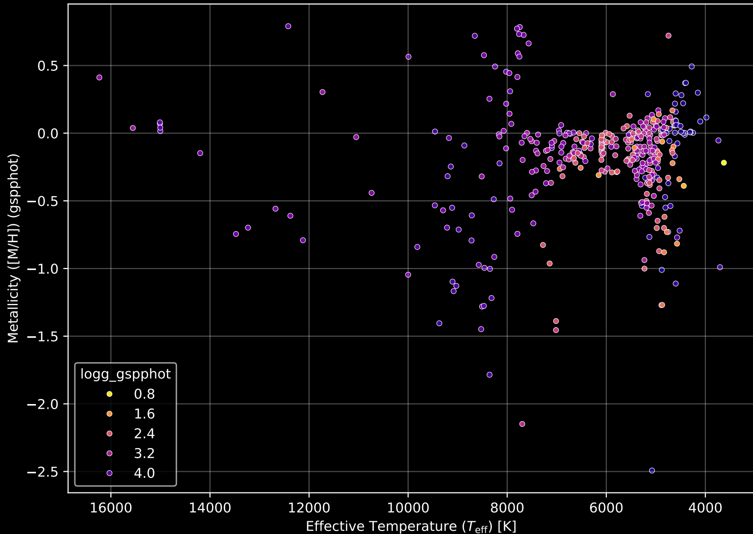
APOGEE DR17 Field: [180+00] Stellar Population Parameters (n= 396)
